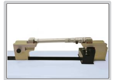
内径千分尺对零或校验
